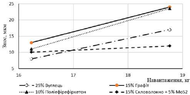
Рис. 3. Лінійний знос композиційних матеріалів на основі тefлону в умовах мащення оливою
