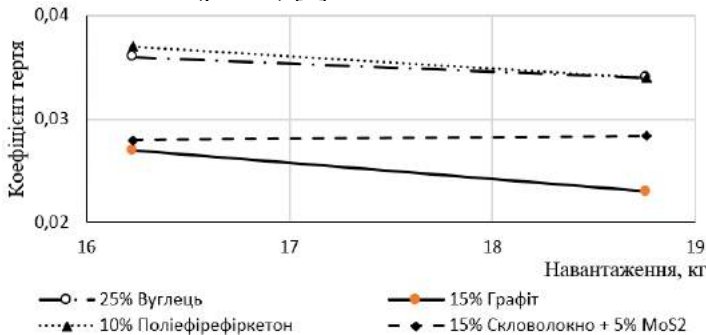
Рис. 4. Зміна коефіцієнту тертя для зразків композиційних матеріалів на основі тefлону в умовах мащення оливою
