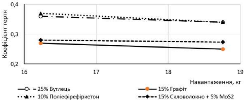
Рис. 2. Кінетика зміни коефіцієнту тертя при збільшенні навантаження для композиційних матеріалів на основі тefлону без використання мастильного матеріалу
