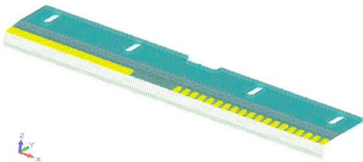
Рис. 4. Модель ріжучого леза ножа подрібнюючого барабану комбайна з дискретним покриттям із карбиду вольфраму ВК8 нанесеним методом електроіскрового легування
